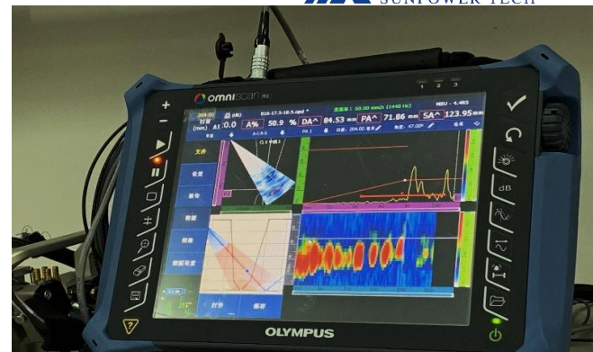
TOFD+PAUT
